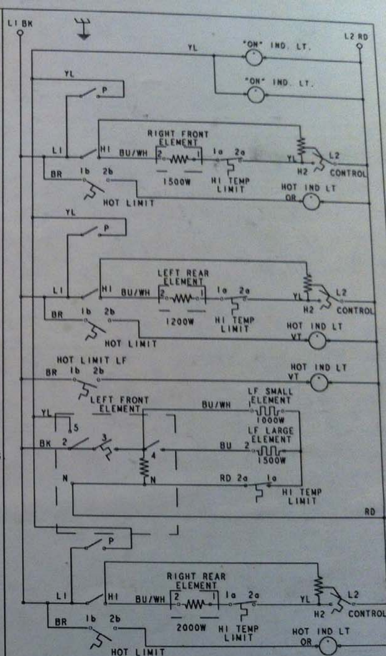
WIRING SCHEMATIC
