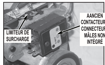
FIGURE 2A (MOTEUR DÉFECTUEUX)
