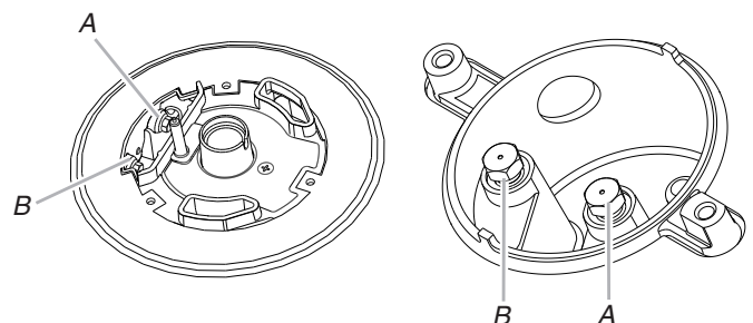
A. Inner orifice spud B. Outer orifice spud
